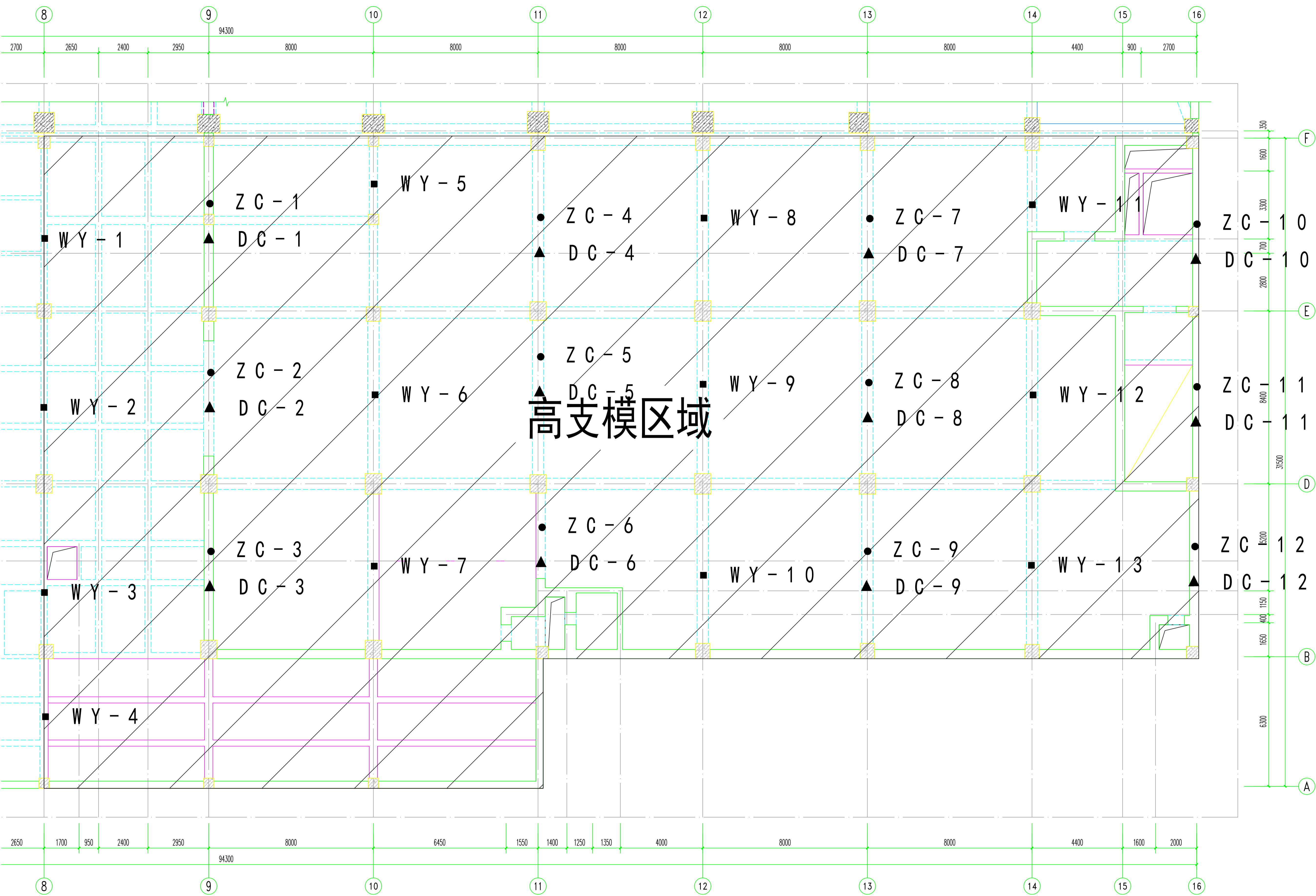
负二层A区监测平面布置图
